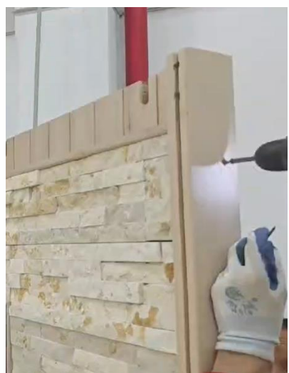
7. Screw the slats
