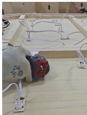
15. Vijcima pričvrstite stropne ploče zajedno i uzduž rubova
