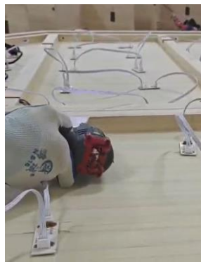
15. Privijačite stropni plošči med sabo in po robovih
