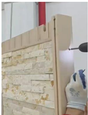
7. Zašrafite letve
